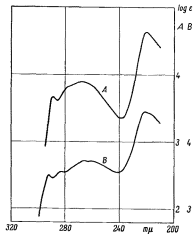
Abb. 2. A: Psilocybin } in Methanol B: Psilocin }
